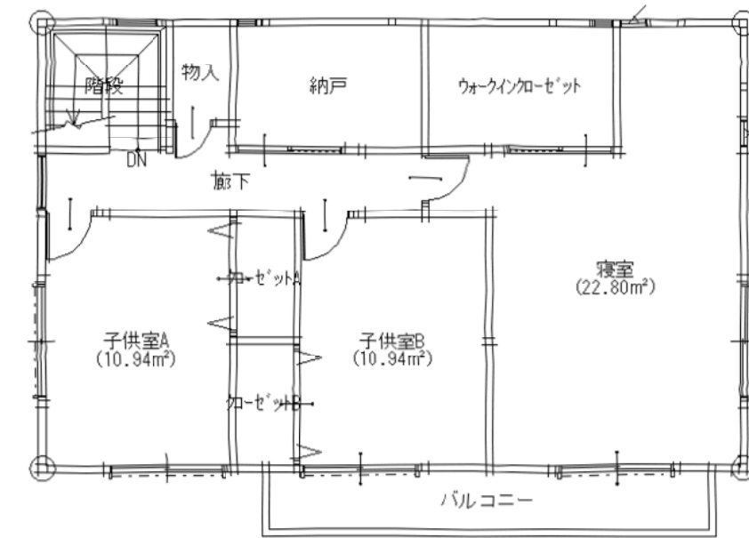
2階平面図
